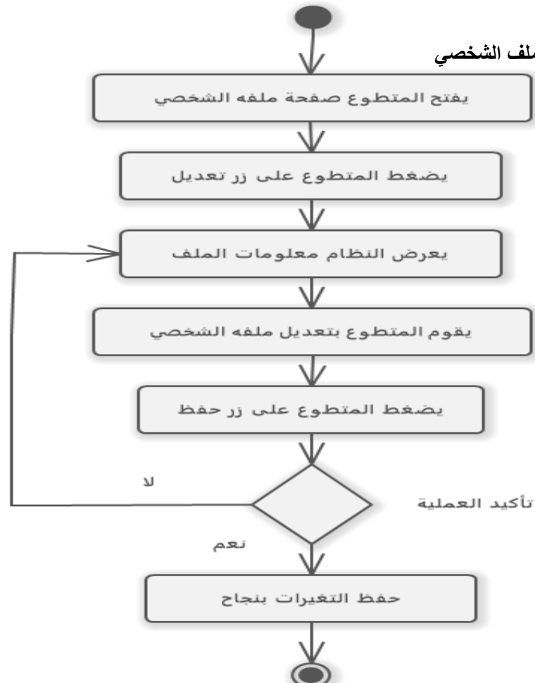
رسم توضيحي 73-مخطط النشاط تعديل الملف الشخصي
