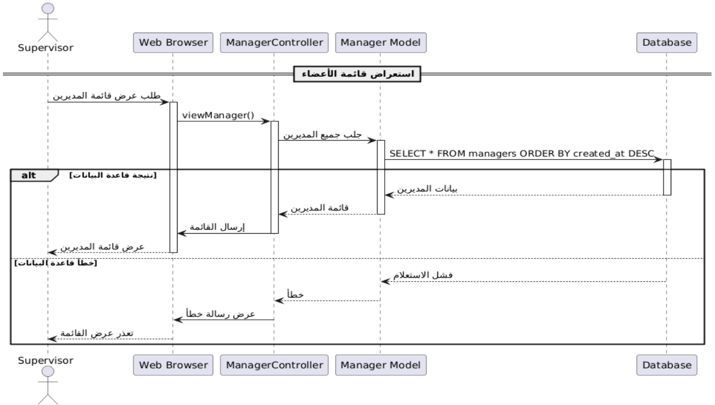
رسم توضيحي 94- مخطط التسلسل استعراض قائمة الاعضاء
