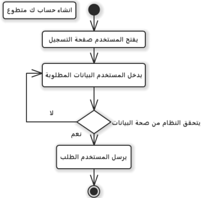
رسم توضيحي 78- مخطط النشاط انشاء حساب تطوع
