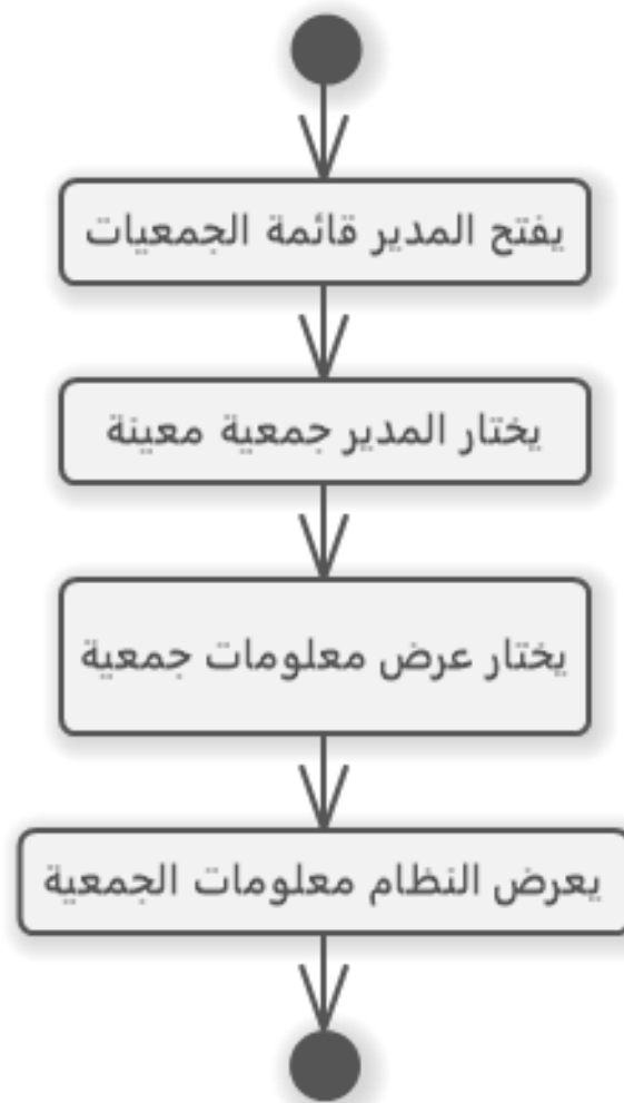
رسم توضيحي 37- مخطط النشاط عرض معلومات جمعية
