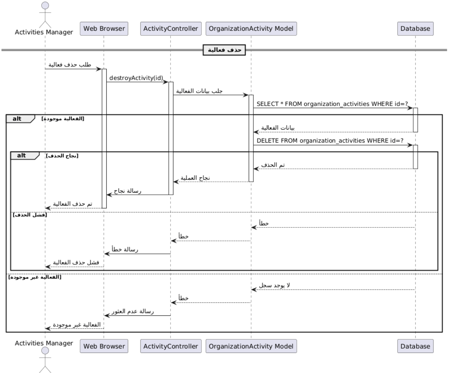
رسم توضيحي 101- مخطط التسلسل حذف فعالية
