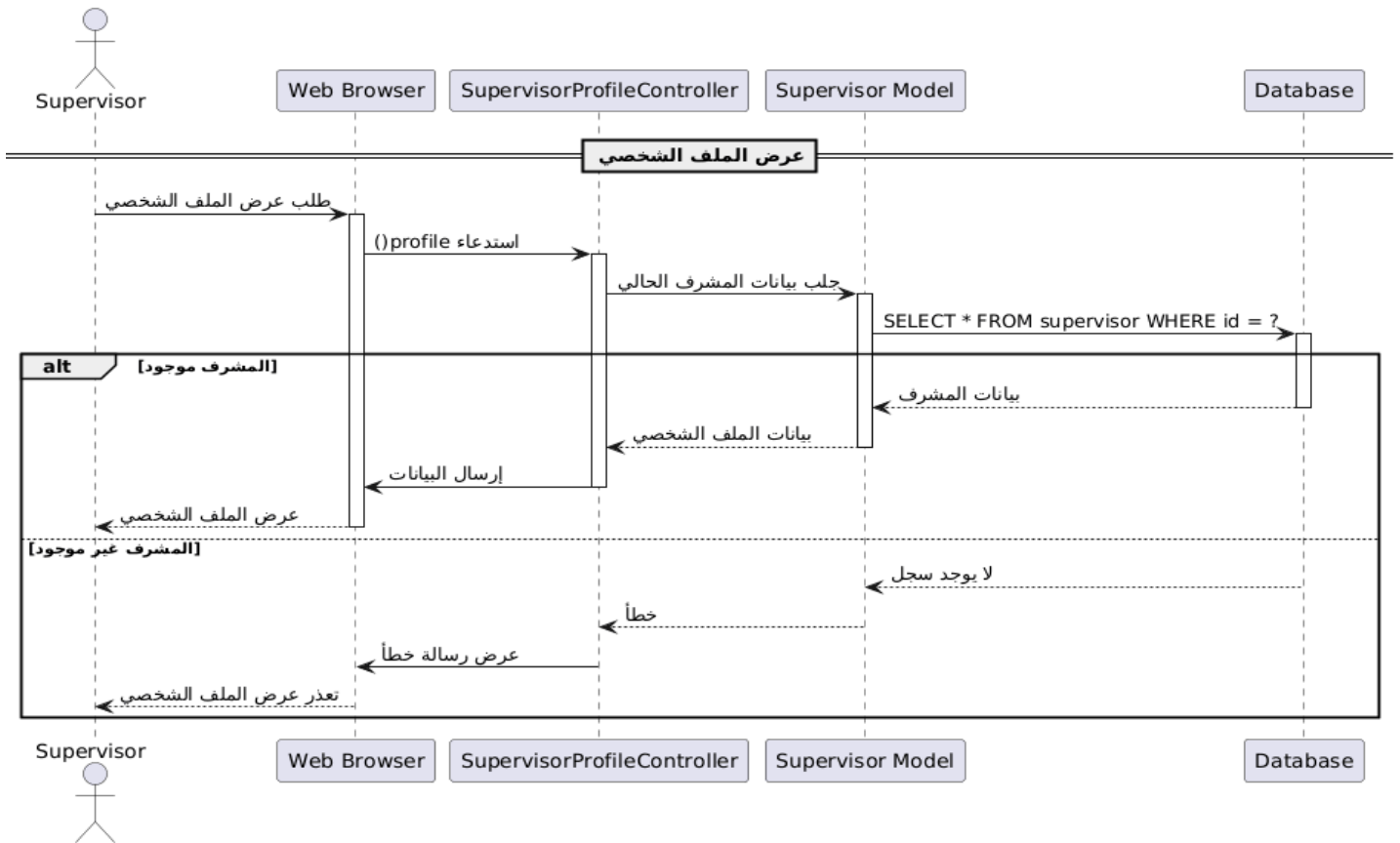
رسم توضيحي 89- مخطط التسلسل عرض الملف الشخصي
