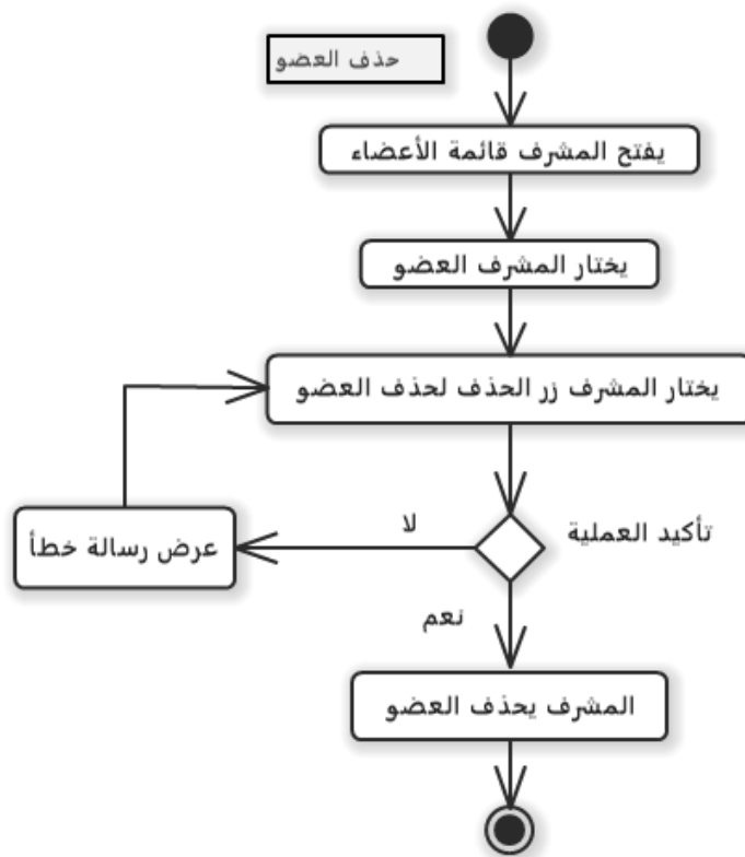
رسم توضيحي 17-مخطط النشاط حذف عضو
