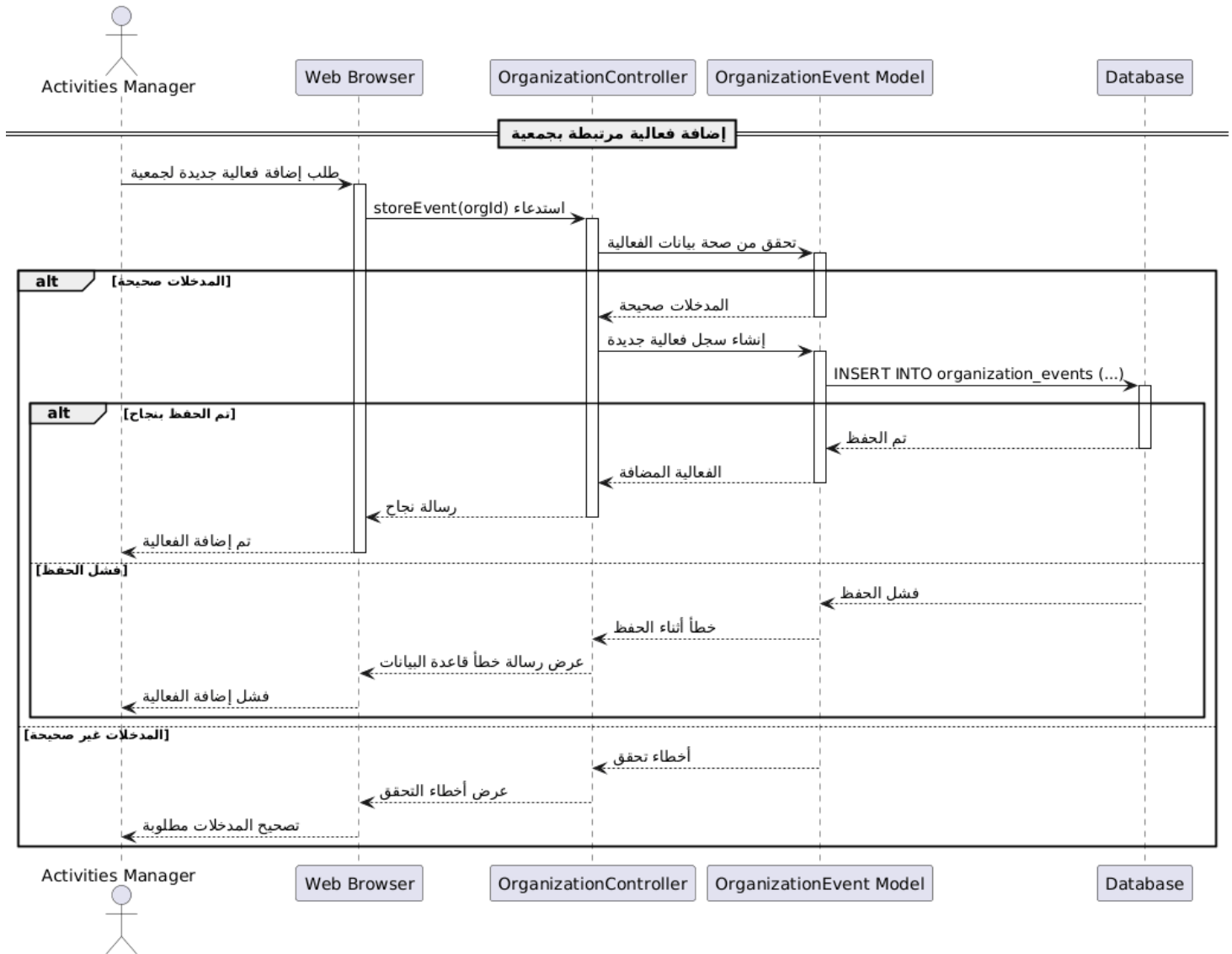
رسم توضيحي 118- مخطط التسلسل إضافة فعالية مرتبطة بجمعية
