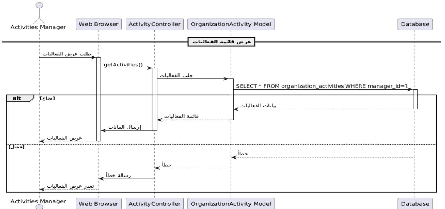
رسم توضيحي 103- مخطط التسلسل استعراض قائمة الفعاليات
