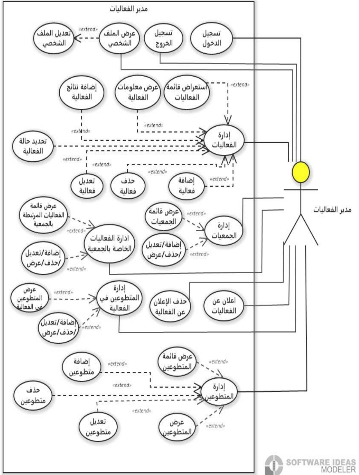
رسم توضيحي 7- Use Case Diagram (مدير الفعاليات)
