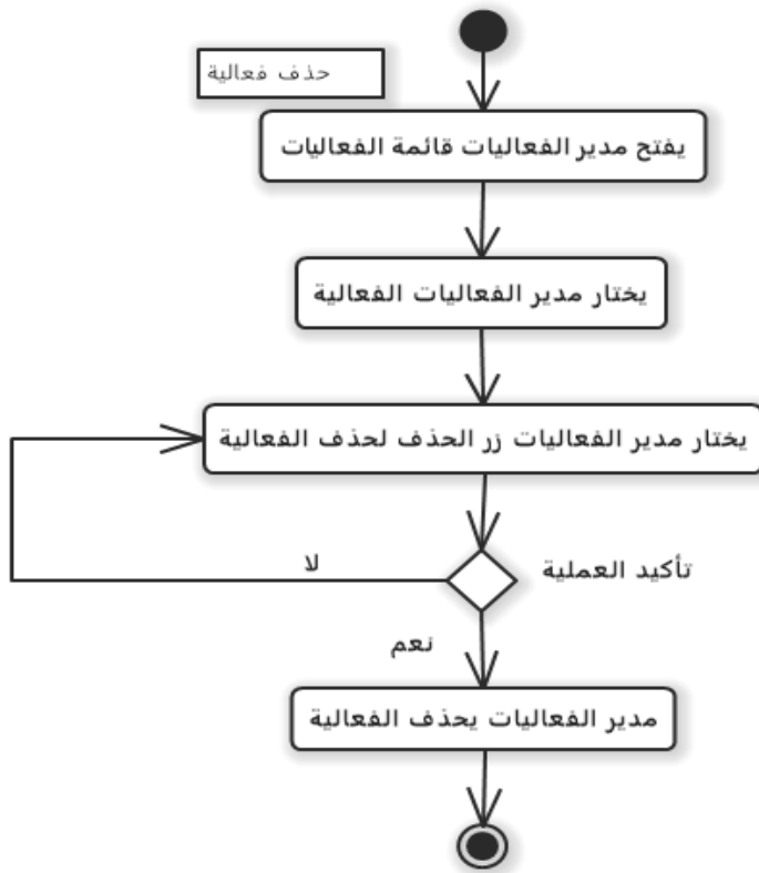
رسم توضيحي 25- مخطط النشاط حذف فعالية
