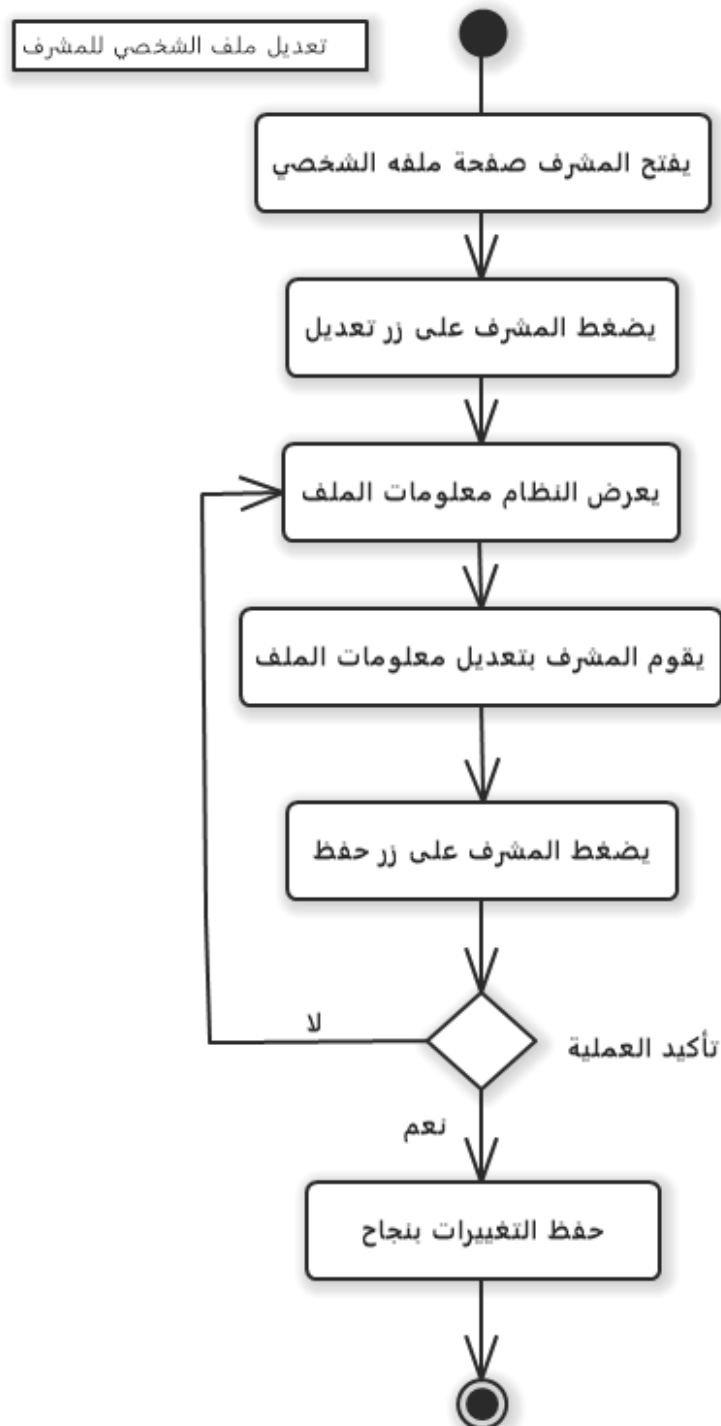
رسم توضيحي 28- مخطط النشاط تعديل الملف الشخصي
