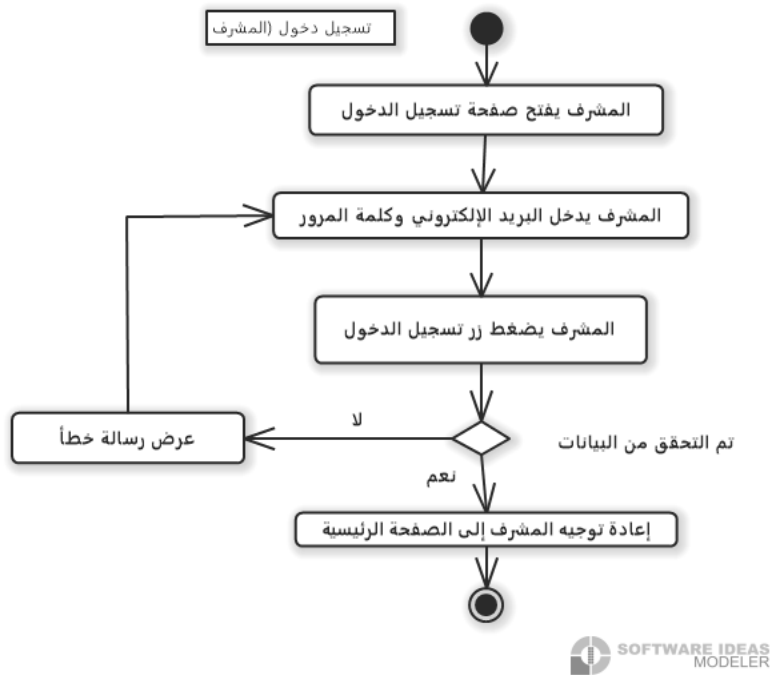
رسم توضيحي 12- مخطط النشاط تسجيل الدخول
