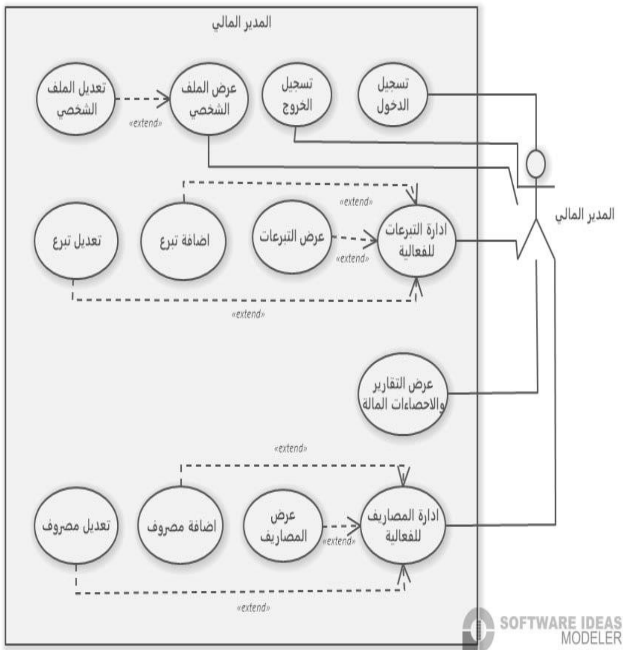
رسم توضيحي 8- Use Case Diagrams (المدير المالي)
