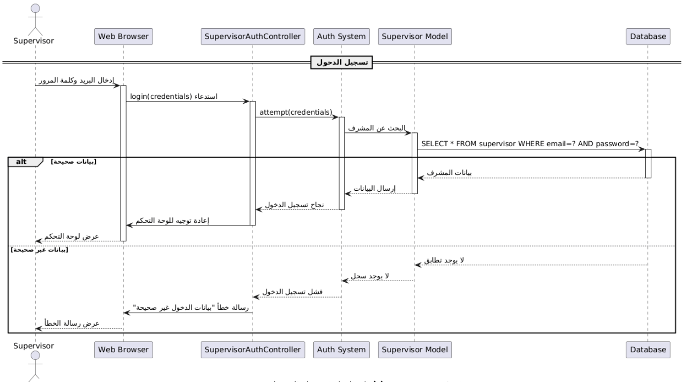
رسم توضيحي 87- مخطط التسلسل تسجيل الدخول
