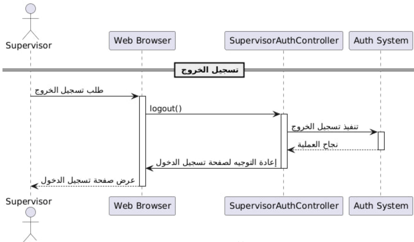
رسم توضيحي 88- مخطط التسلسل تسجيل الخروج
