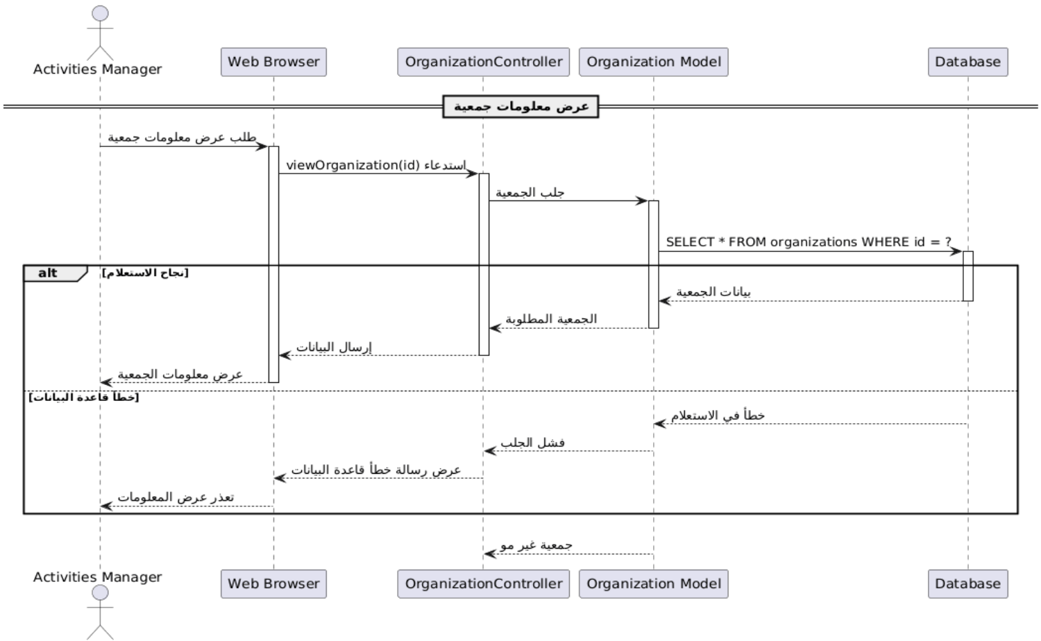
رسم توضيحي 113- مخطط التسلسل عرض معلومات جمعية
