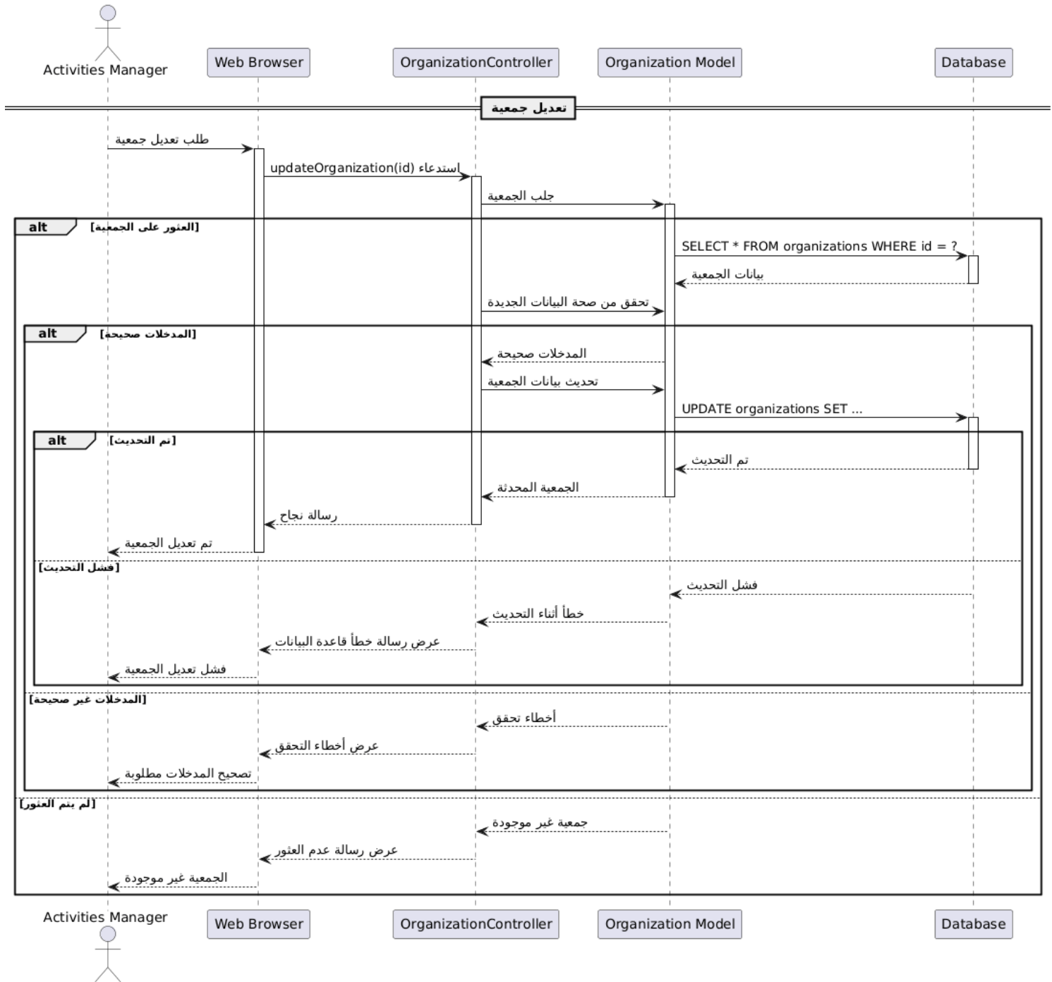
رسم توضيحي 114- مخطط التسلسل تعديل معلومات جمعية
