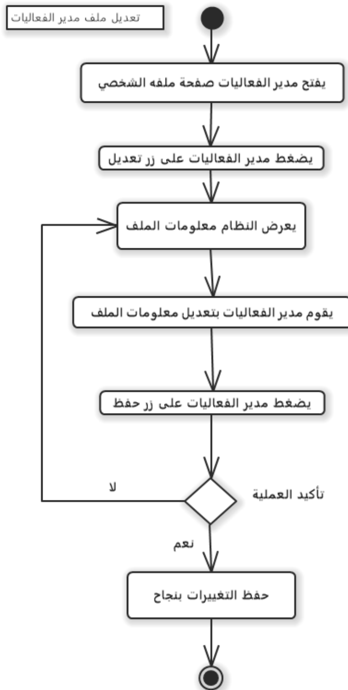
رسم توضيحي 34- مخطط النشاط تعديل الملف الشخصي
