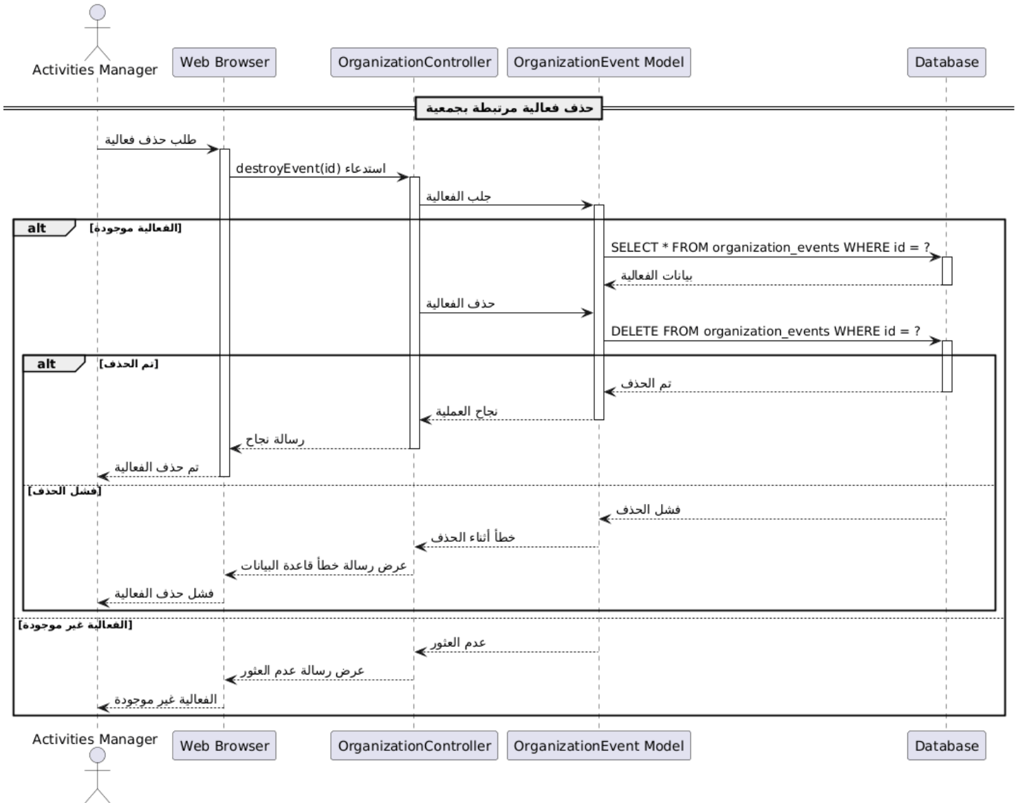
رسم توضيحي 119- مخطط التسلسل حذف فعالية مرتبطة بجمعية
