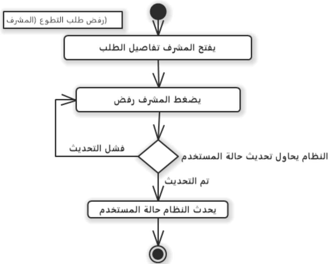
رسم توضيحي 33- مخطط النشاط رفض طلب التطوع
