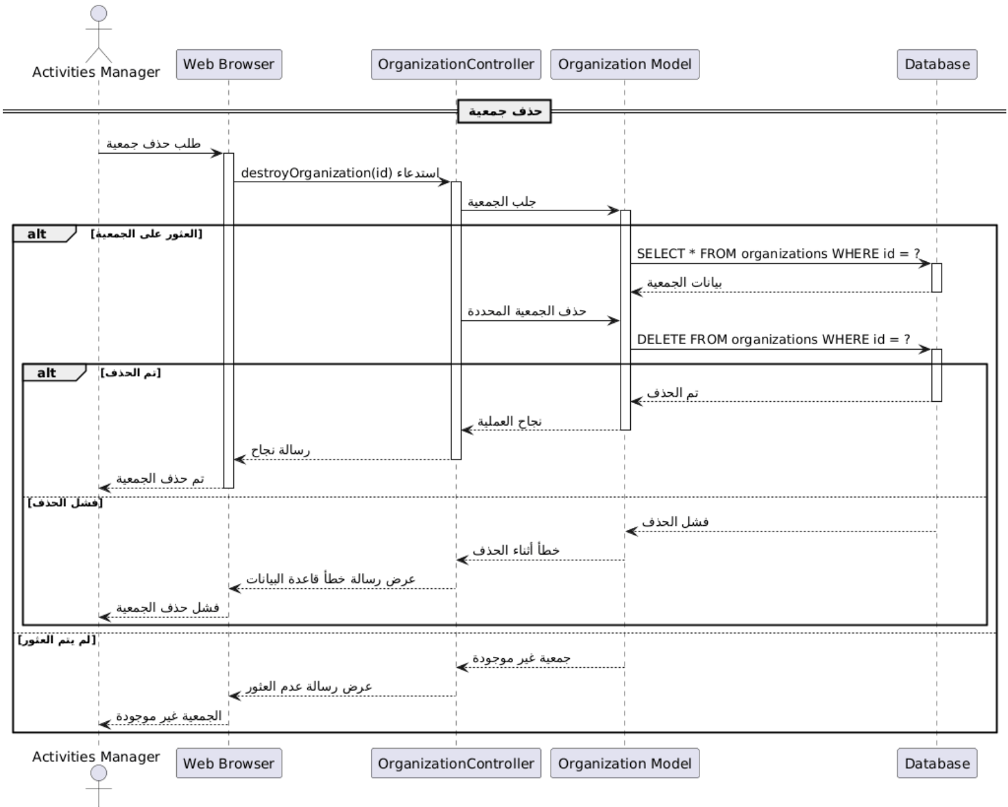
رسم توضيحي 115- مخطط التسلسل حذف جمعية
