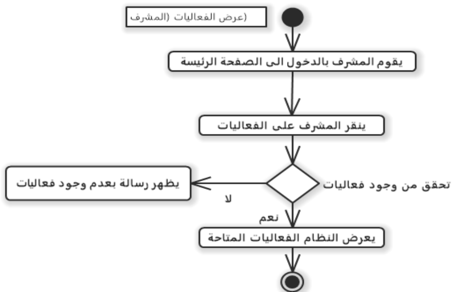
رسم توضيحي 30- مخطط النشاط عرض الفعاليات
