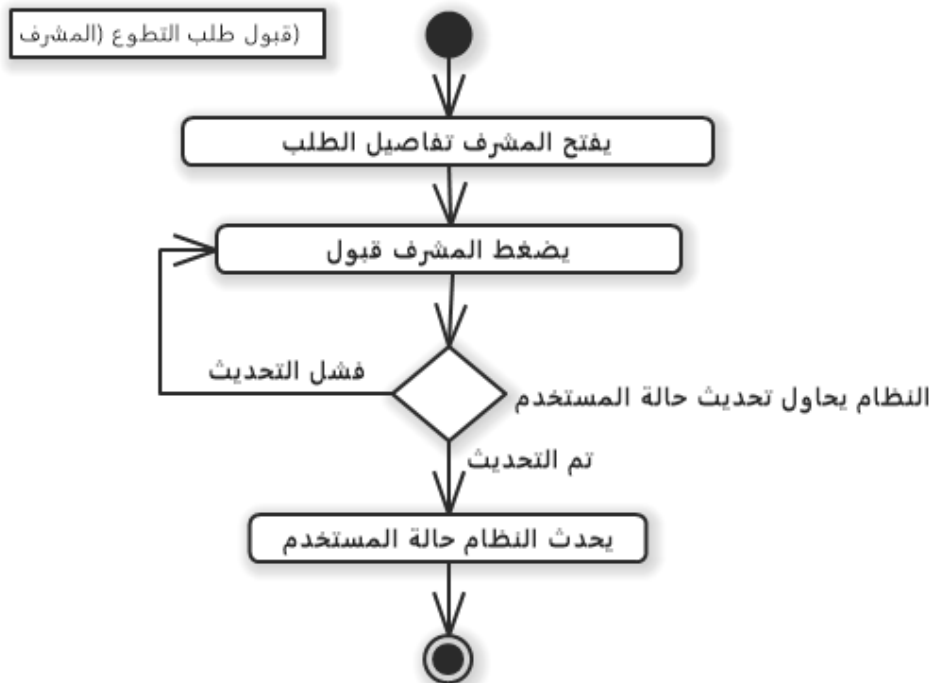
رسم توضيحي 32- مخطط النشاط قبول طلب التطوع
