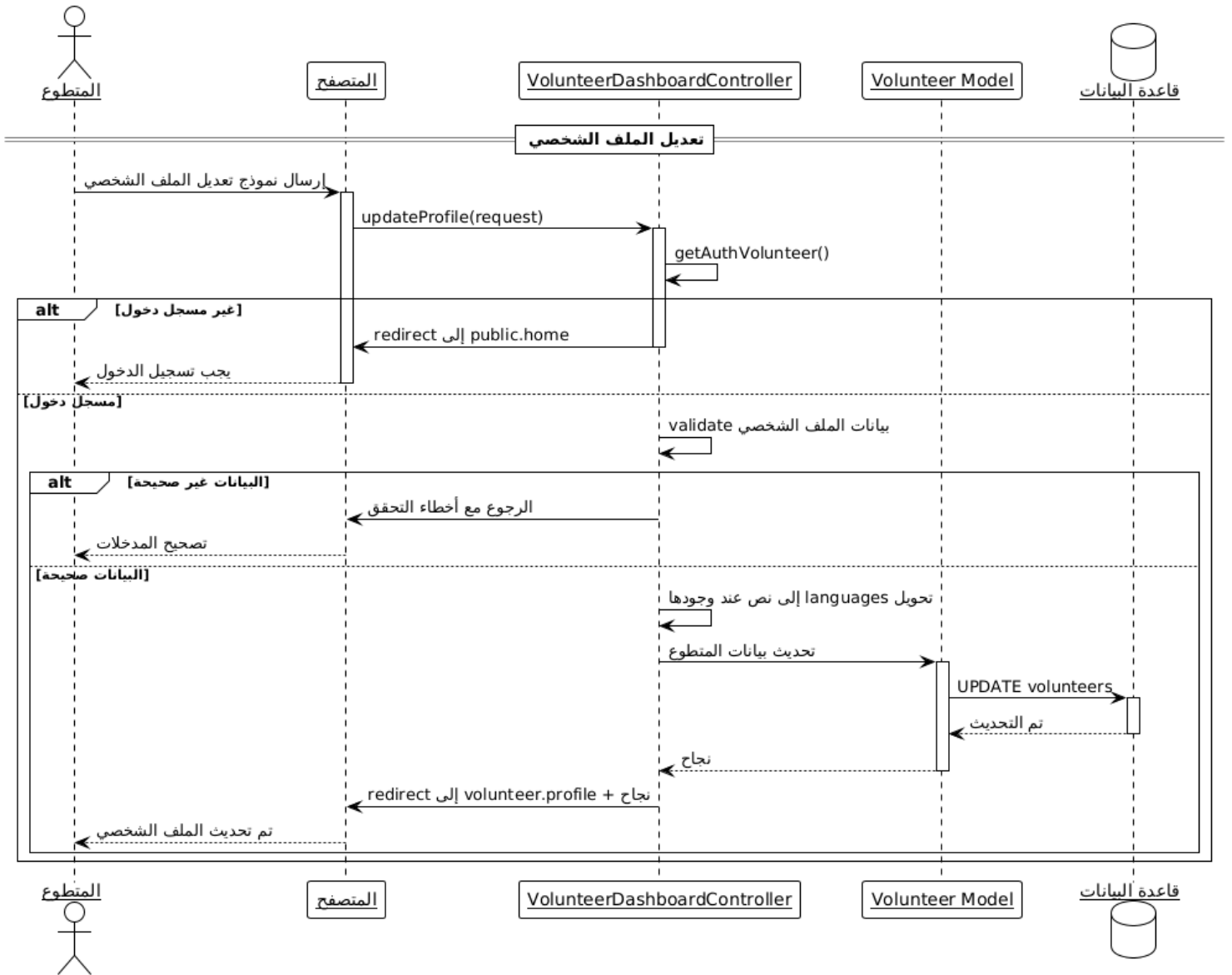
رسم توضيحي 149-مخطط التسلسل تعديل الملف الشخصي
