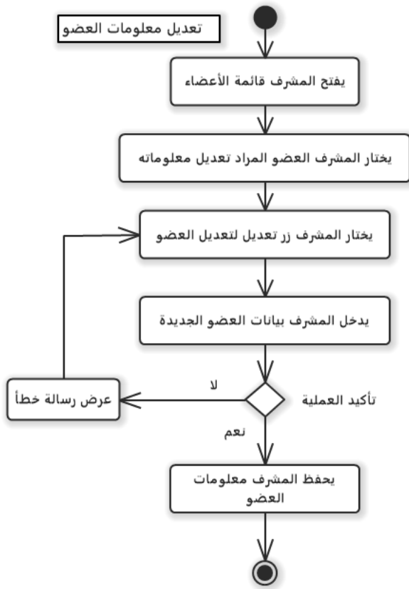
رسم توضيحي 16-مخطط النشاط تعديل معلومات عضو
