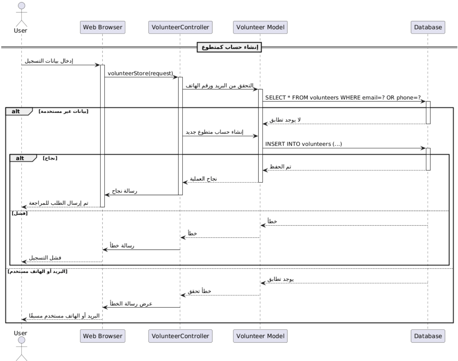
رسم توضيحي 154- مخطط التسلسل انشاء حساب كمتطوع
