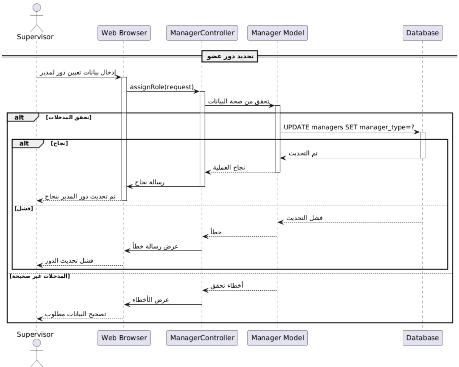
رسم توضيحي 95- مخطط التسلسل تحديد دور الاعضاء
