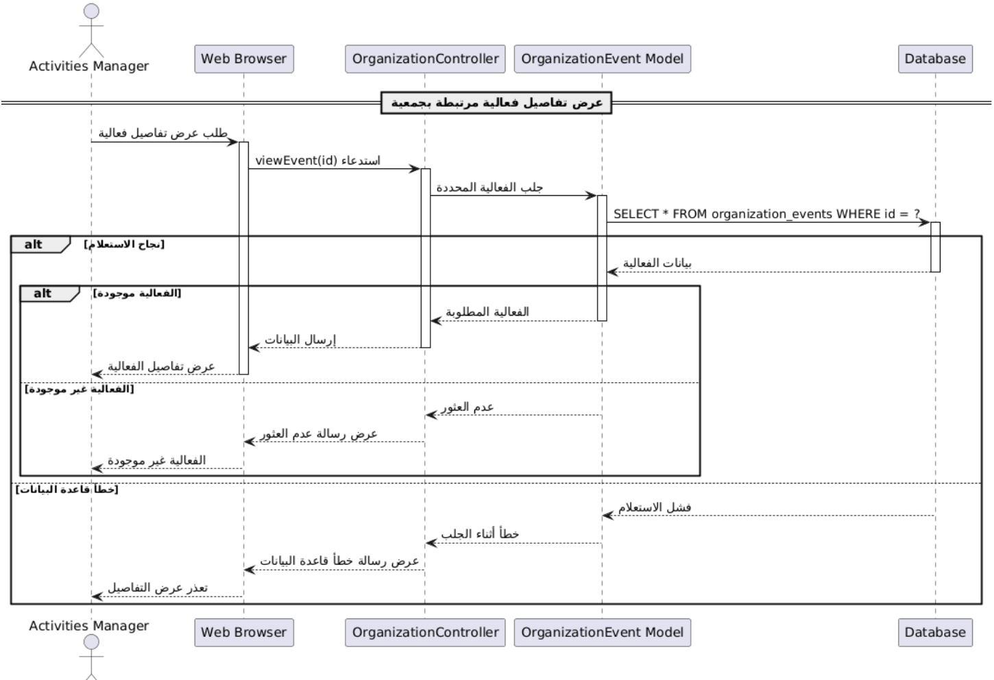
رسم توضيحي 117- مخطط التسلسل عرض معلومات فعالية مرتبطة بجمعية
