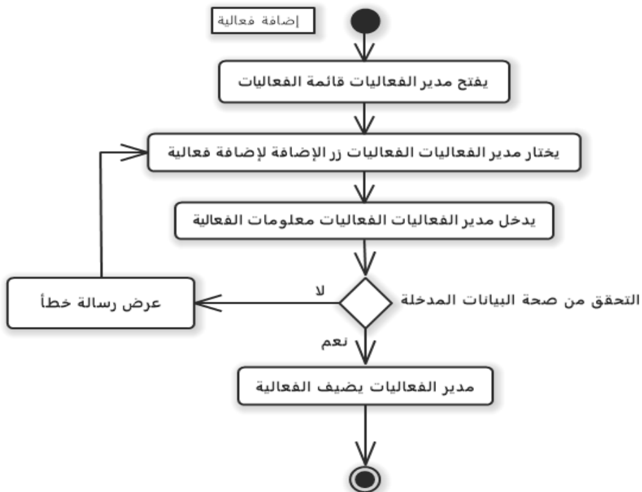
رسم توضيحي 23-مخطط النشاط إضافة فعالية
