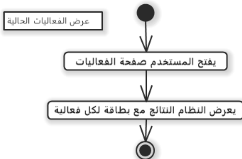
رسم توضيحي 79- مخطط النشاط عرض الفعاليات الحالية
