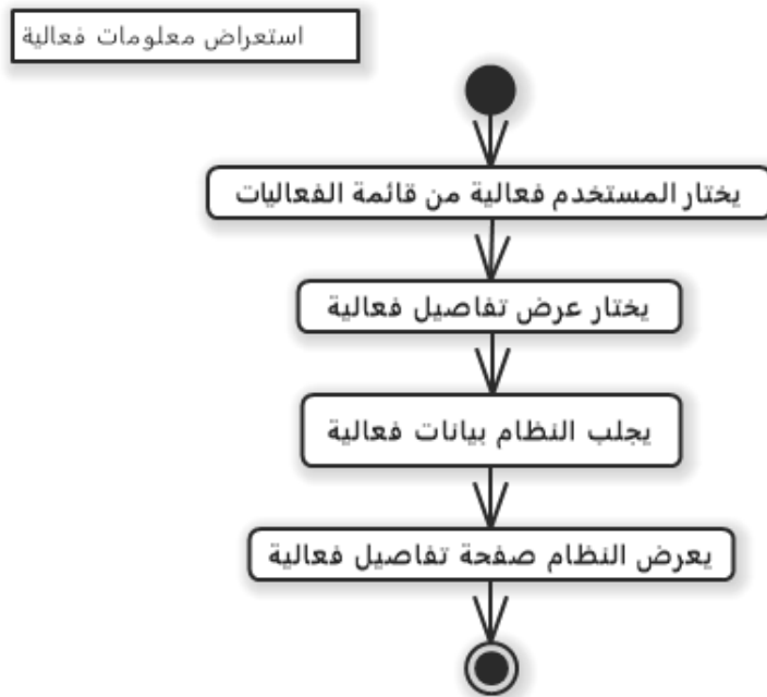
رسم توضيحي 80- مخطط النشاط استعراض معلومات فعالية
