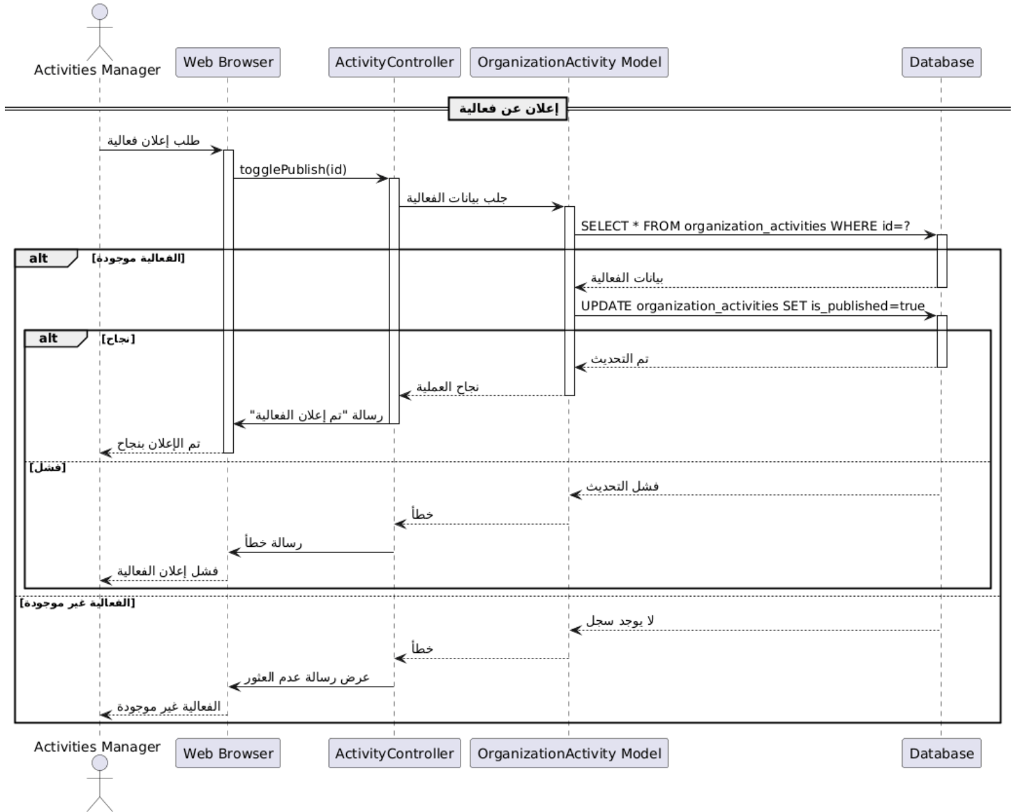
رسم توضيحي 121- مخطط التسلسل اعلان عن فعالية
