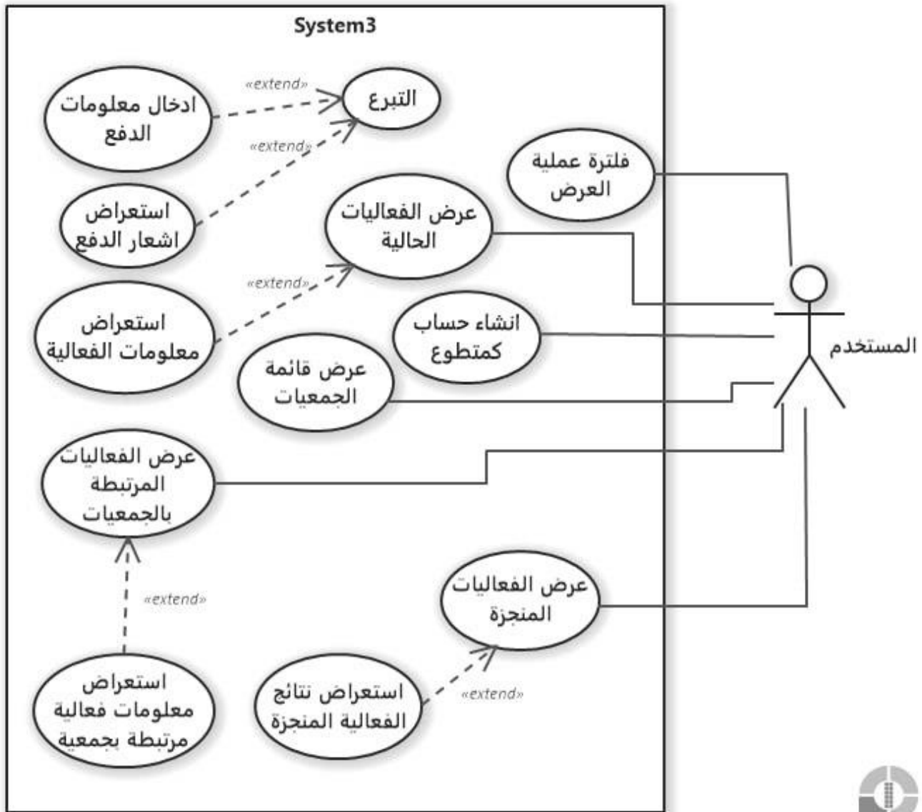
رسم توضيحي 10- Use Case Diagrams (المستخدم)
