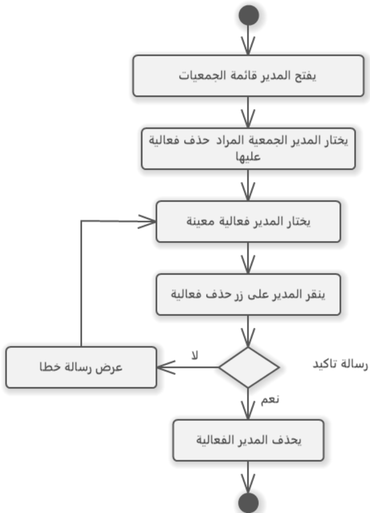
رسم توضيحي 43- مخطط النشاط حذف فعالية مرتبطة بجمعية
