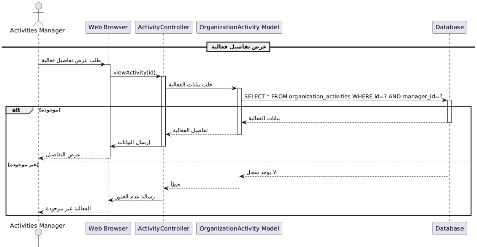
رسم توضيحي 102- مخطط التسلسل عرض معلومات فعالية
