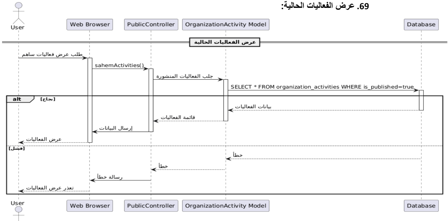
رسم توضيحي 155-مخطط التسلسل عرض الفعاليات الحالية
