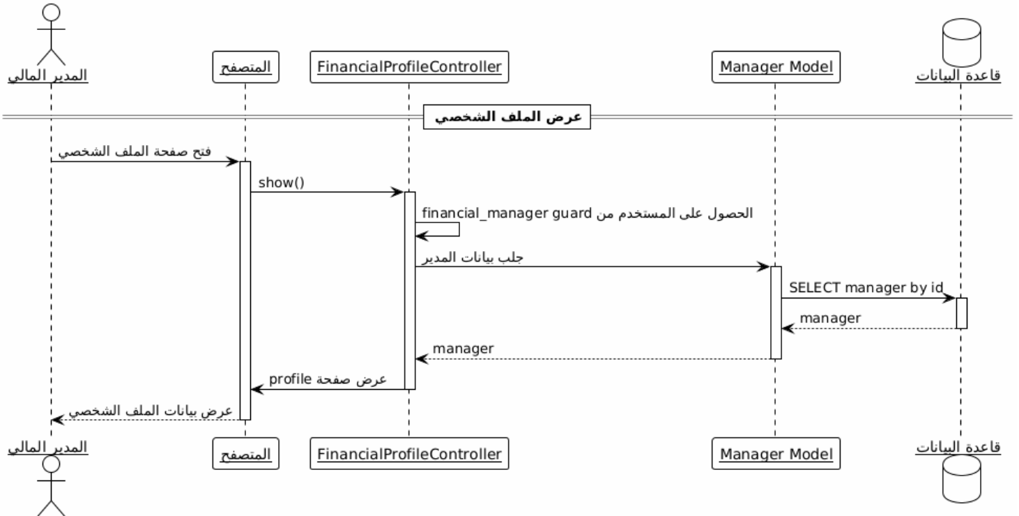
رسم توضيحي 137--مخطط التسلسل عرض الملف الشخصي
