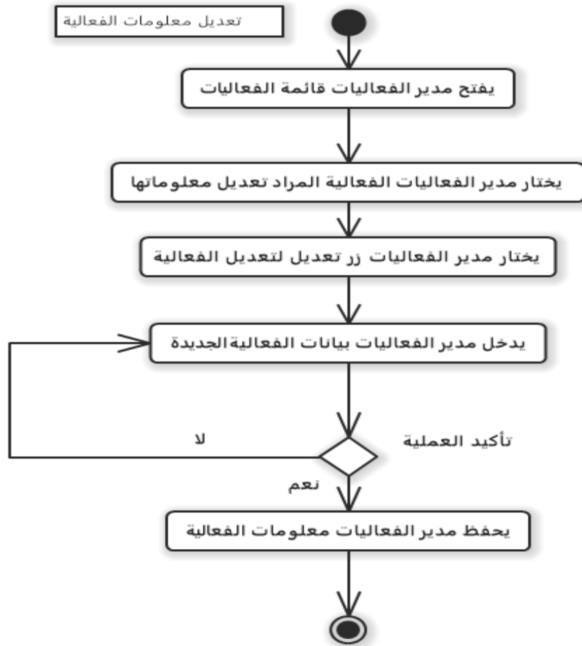
رسم توضيحي 24-مخطط النشاط تعديل معلومات الفعالية
