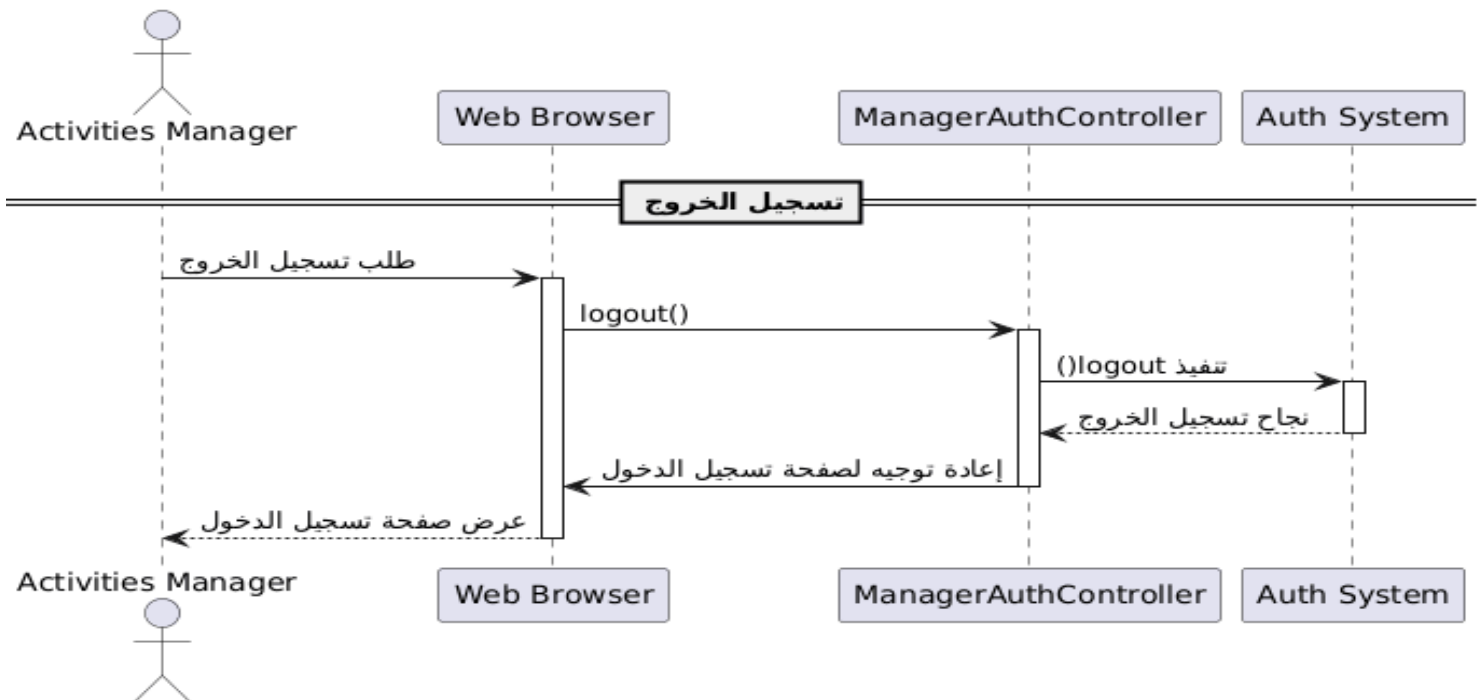
رسم توضيحي 97- مخطط التسلسل تسجيل الخروج
