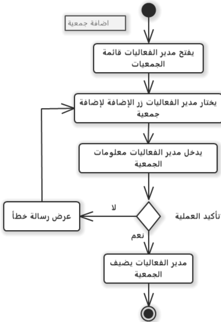
رسم توضيحي 36- مخطط النشاط اضافة جمعية
