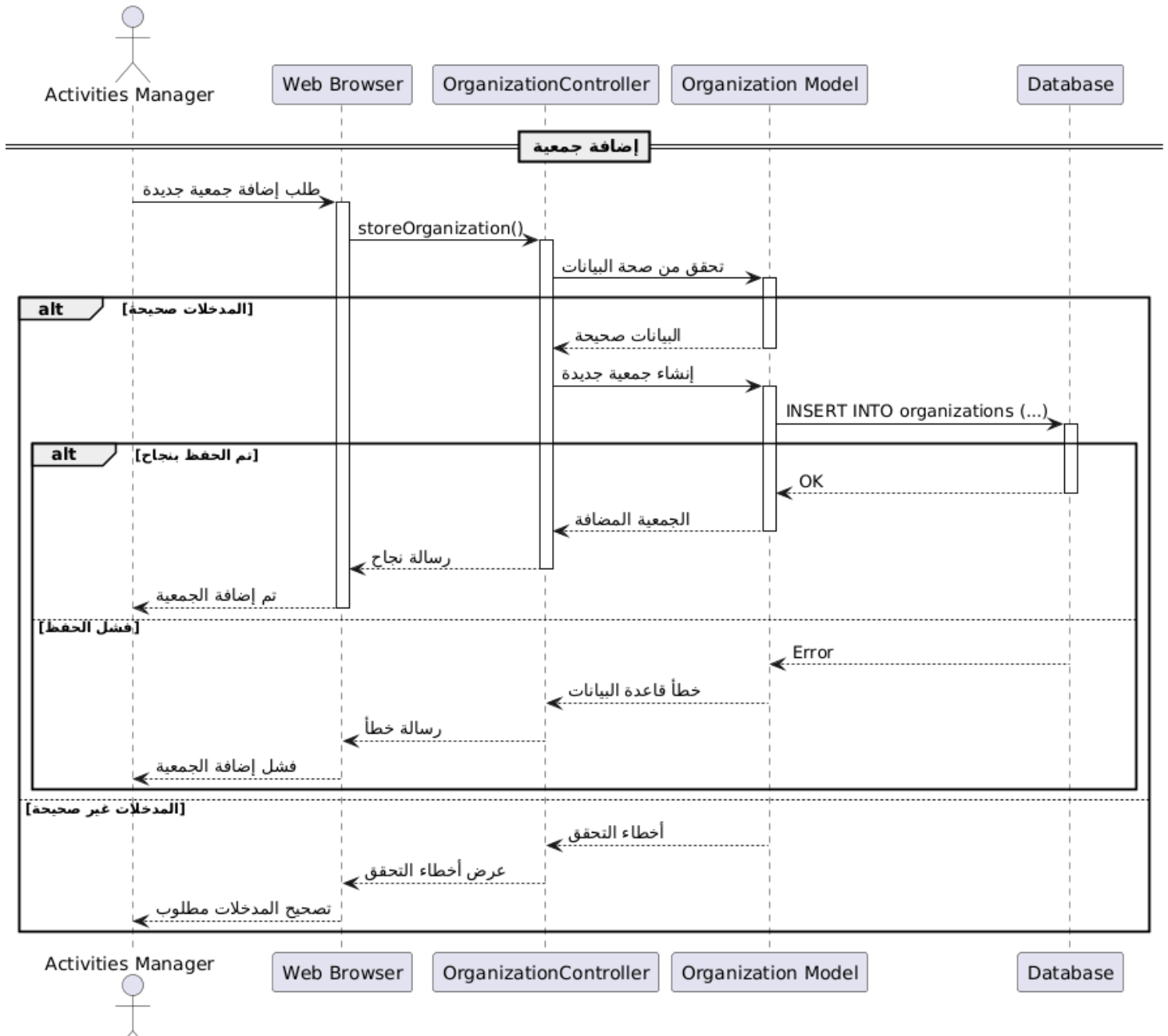
رسم توضيحي 112- مخطط التسلسل إضافة جمعية
