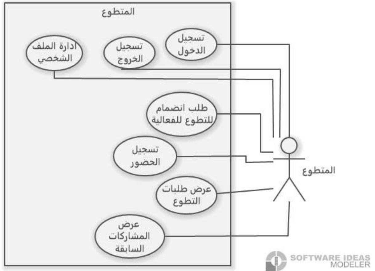
رسم توضيحي 9-- Use Case Diagrams (المنطوع)
