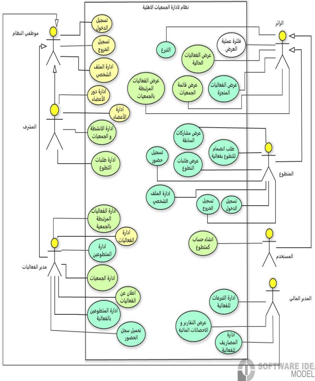
رسم توضيحي 5: (النظام كامل) Use Case Diagrams
