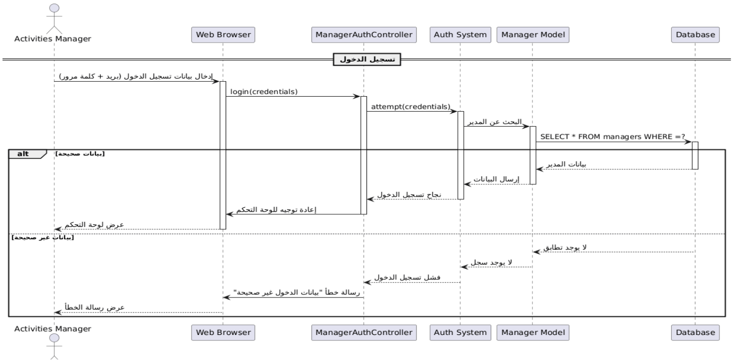
رسم توضيحي 96- مخطط التسلسل تسجيل الدخول
