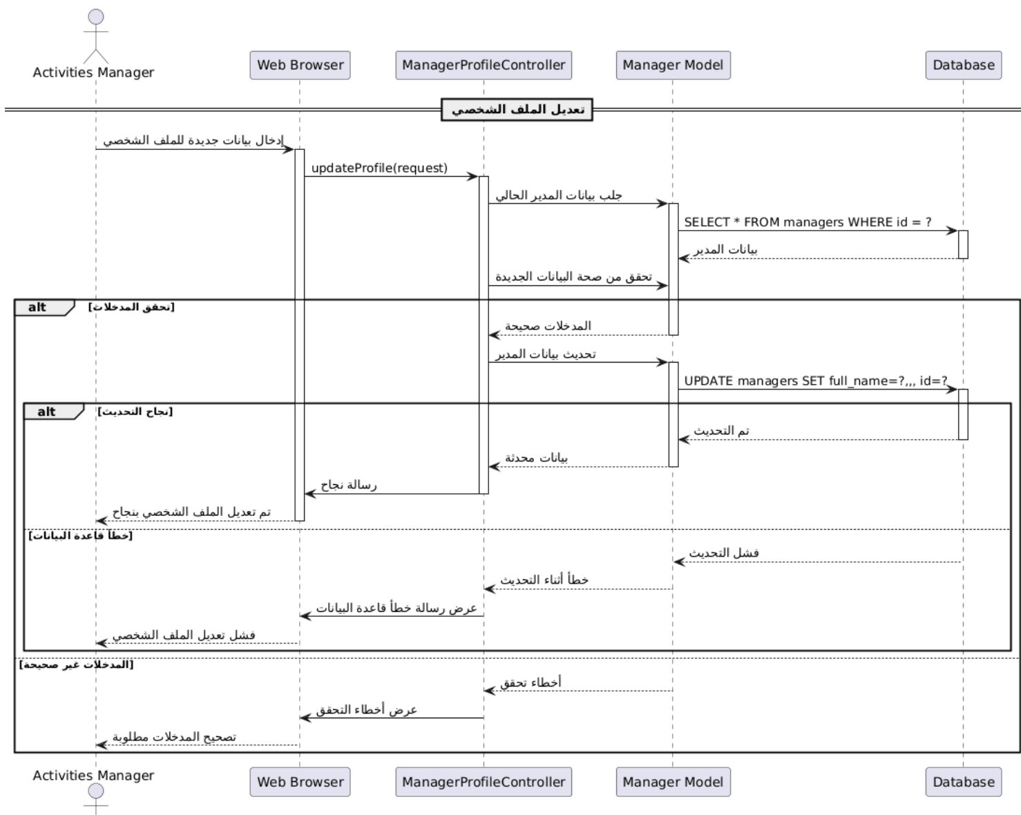
رسم توضيحي 110- مخطط التسلسل تعديل الملف الشخصي
