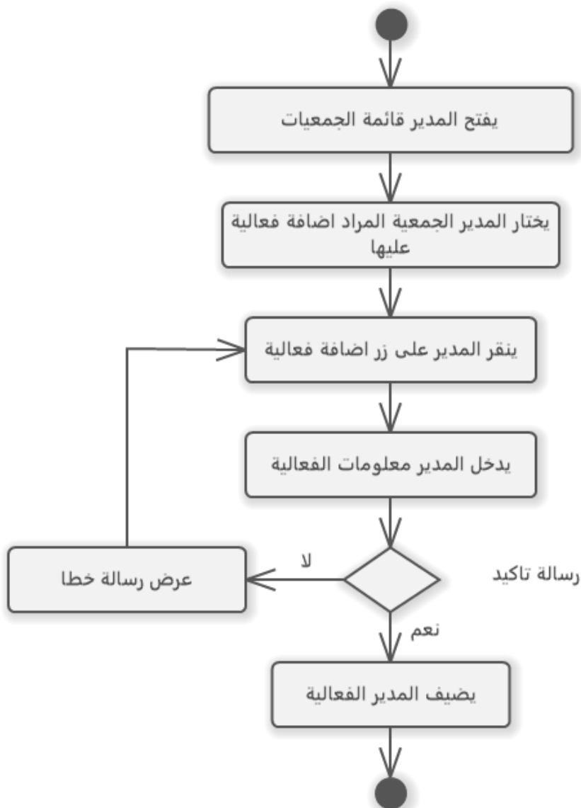
رسم توضيحي 42- مخطط النشاط اضافة فعالية مرتبطة بجمعية
