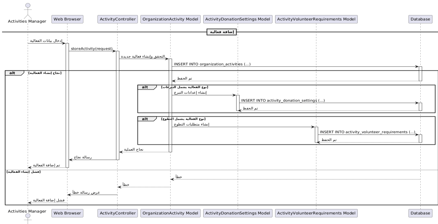
رسم توضيحي 99- مخطط التسلسل إضافة فعالية
