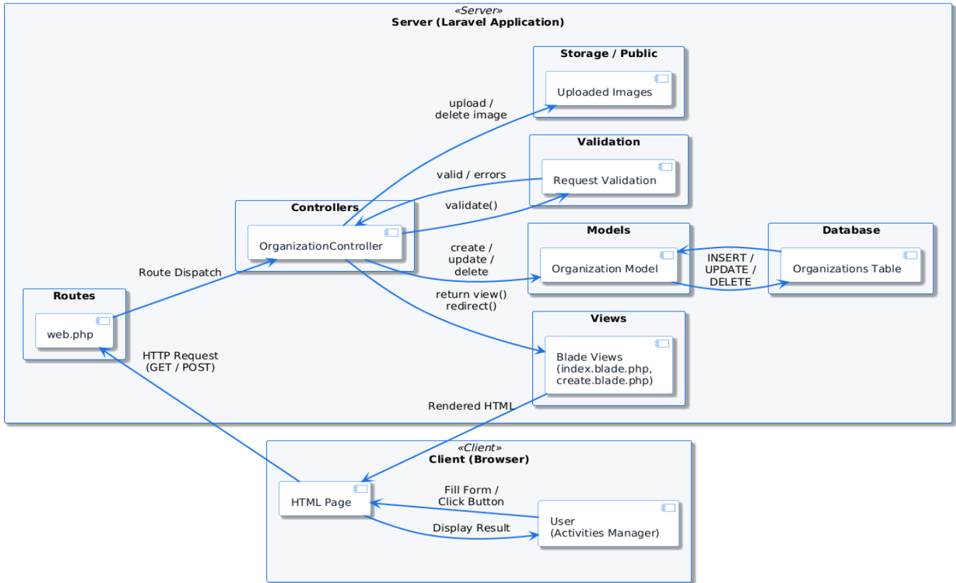
رسم توضيحي 163 - Model-View-Controller
