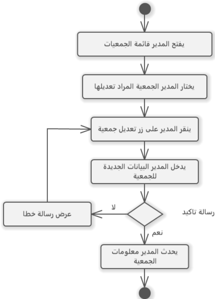
رسم توضيحي 38- مخطط النشاط تعديل معلومات جمعية
