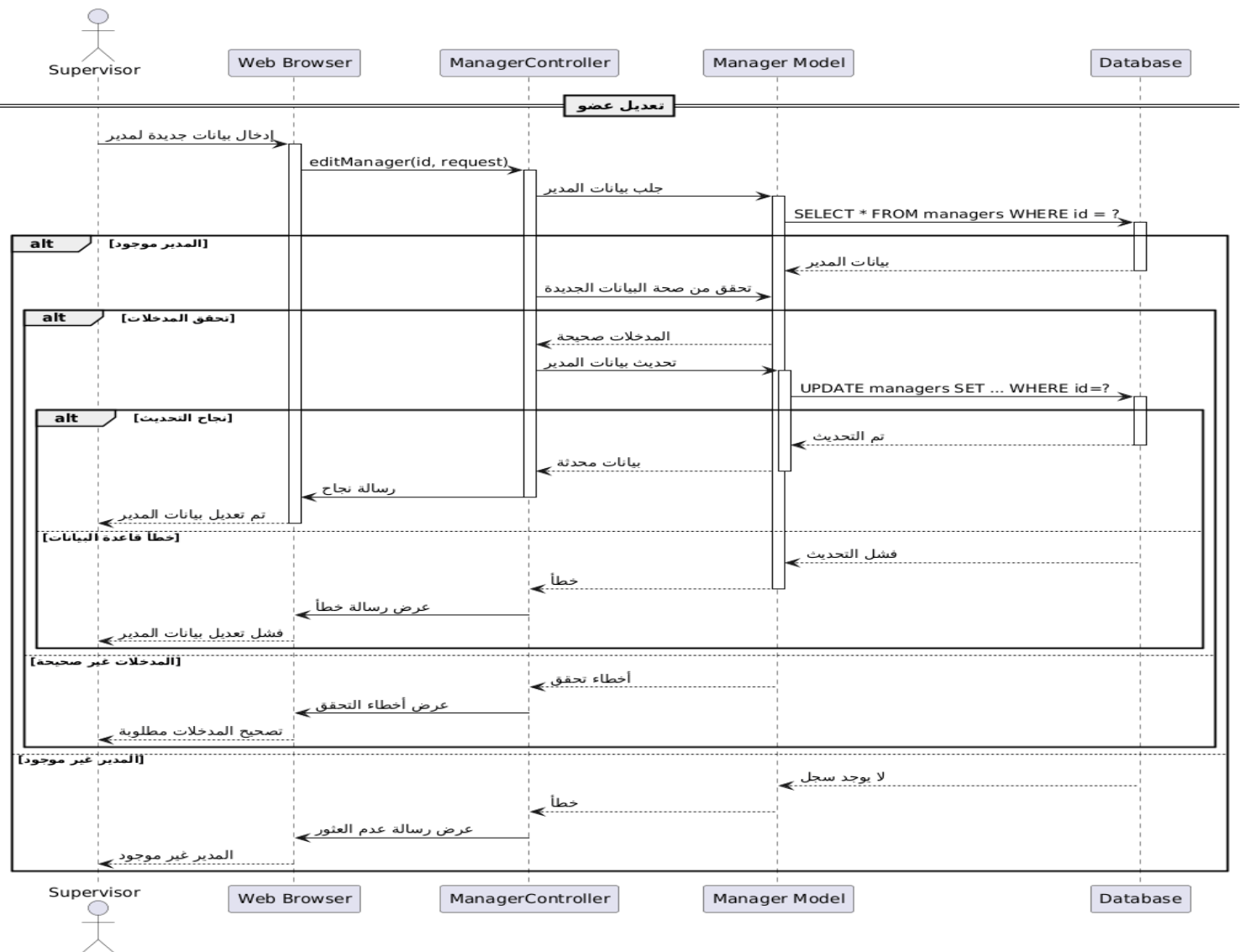
رسم توضيحي 92- مخطط التسلسل تعديل معلومات العضو
