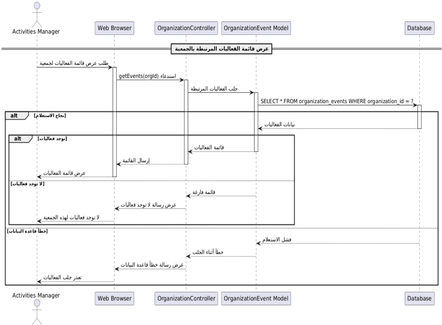
رسم توضيحي 116- مخطط التسلسل عرض قائمة الفعاليات المرتبطة بجمعية
