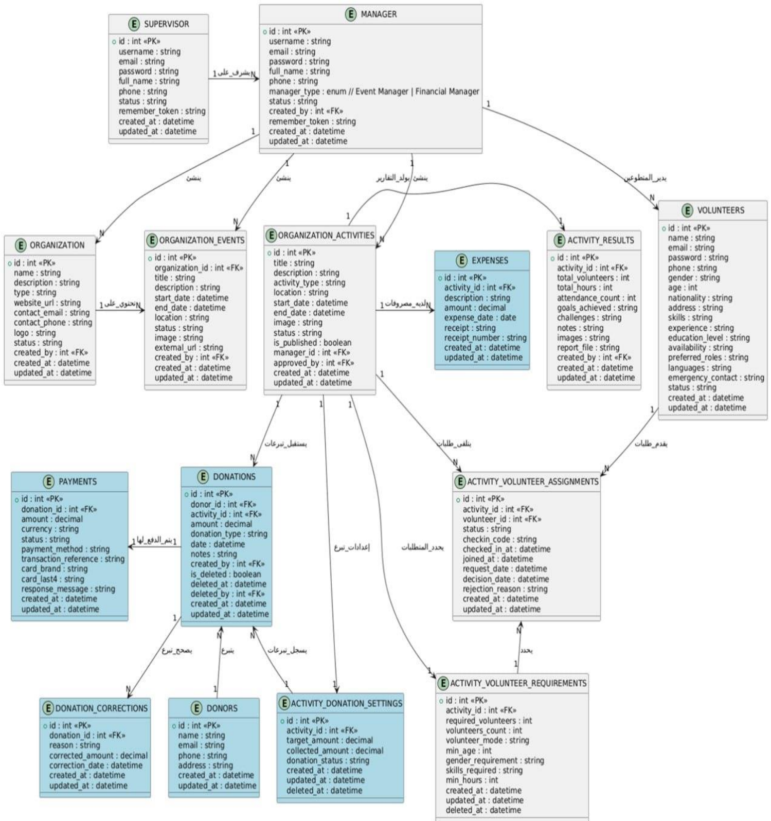
رسم توضيحي 165 - مخطط الجدول (Table Diagram)
