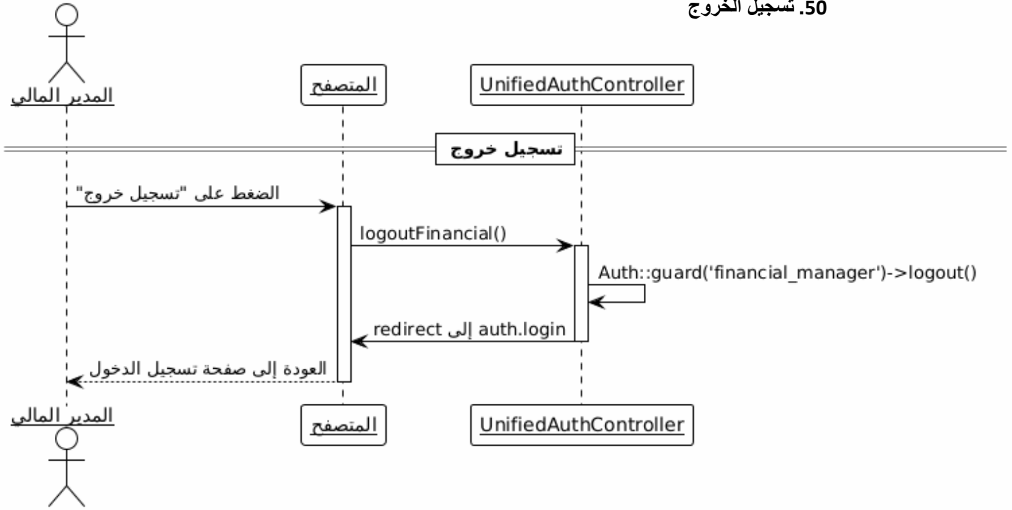
رسم توضيحي 136--مخطط التسلسل تسجيل خروج
