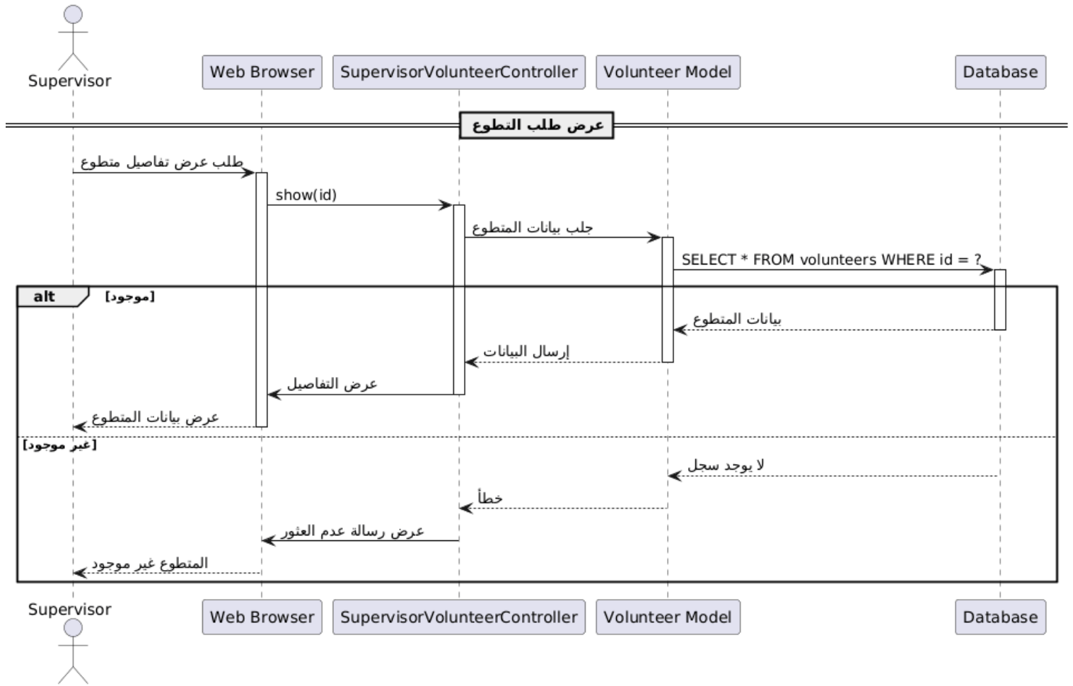
رسم توضيحي 107- مخطط التسلسل عرض طلب التطوع
