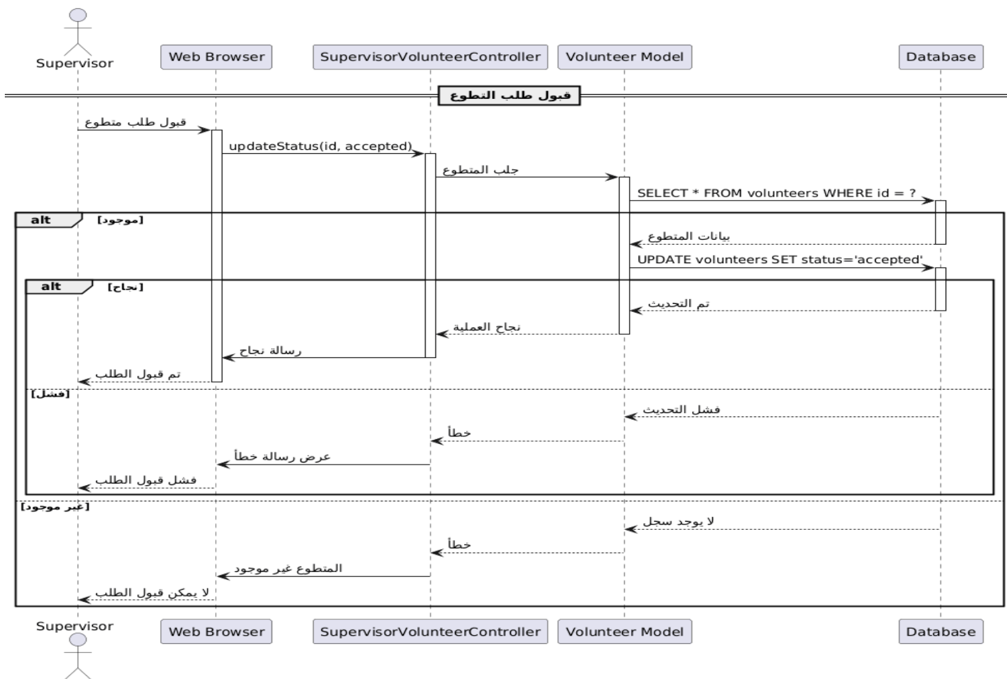
رسم توضيحي 108- مخطط التسلسل قبول طلب التطوع
