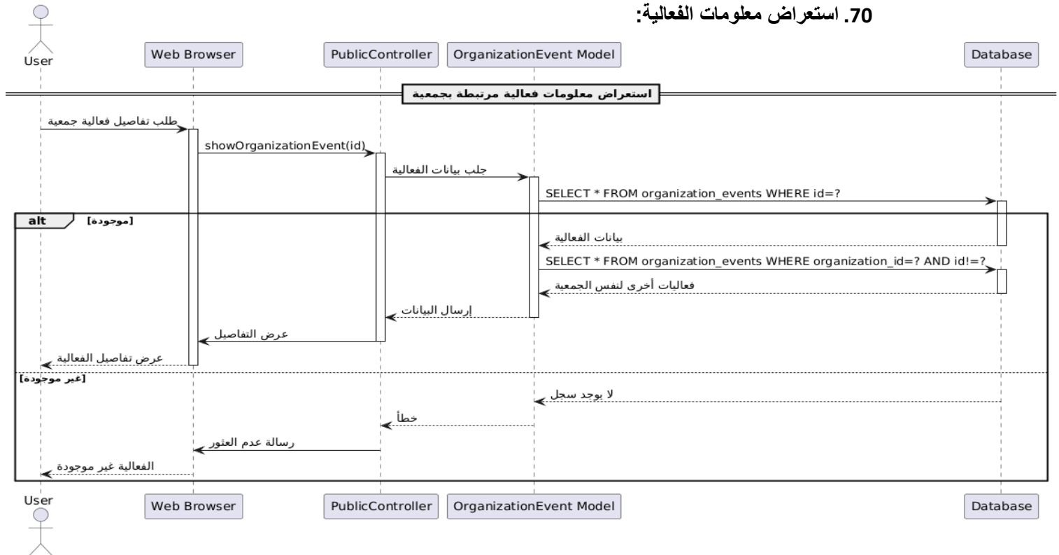
رسم توضيحي 156- مخطط التسلسل استعراض معلومات الفعالية
