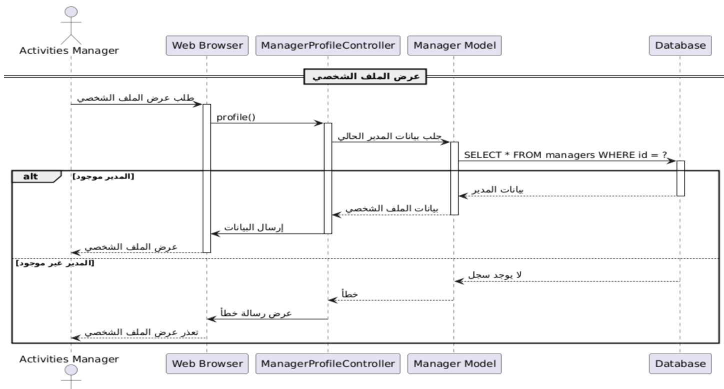
رسم توضيحي 98- مخطط التسلسل عرض الملف الشخصي
