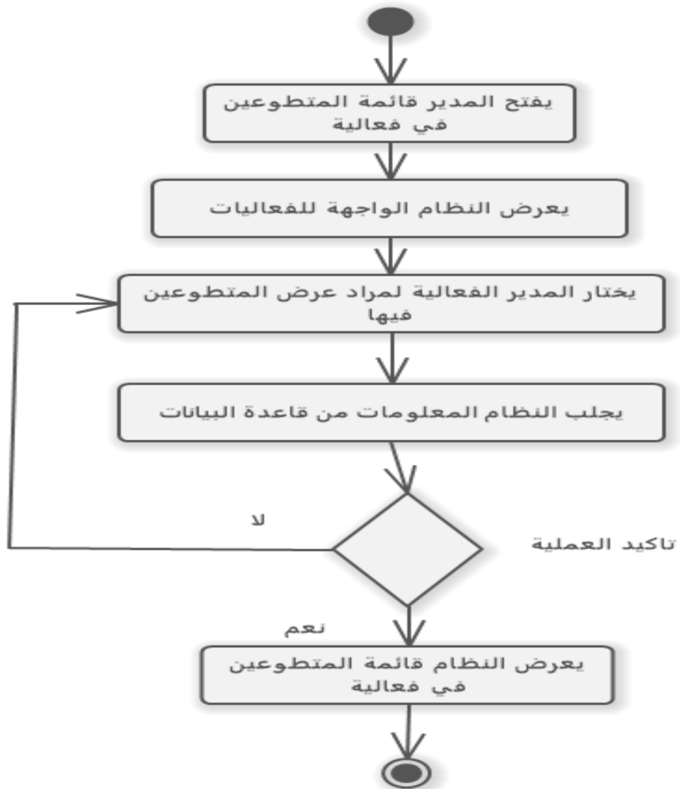
رسم توضيحي 47- مخطط النشاط لعرض المتطوعين في الفعالية
